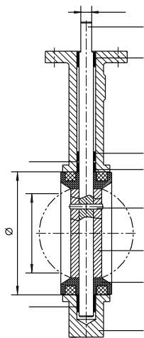
Side View Wafer & Lug Style
